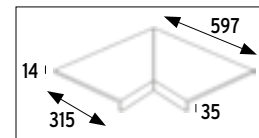
Peldaño recto ingleteado bajo pedido Mitered straight stair tread on demand
