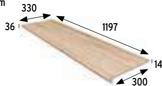
Peldaño redondeado 150* Rounded stair-tread 150
