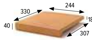
Vierteaguas 25x33 Natural wash 25x33 330x244x40x21 mm
