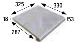
Peldaño redondeado 33 Rounded stair-tread 33 325x330x18 mm
