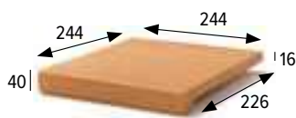
Vierteaguas 25x25 Natural wash 25x25 244x244x40x16 mm
