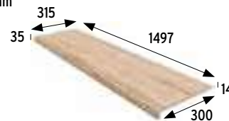
Peldaño recto 180* Straight stair-tread 180
