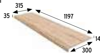
Peldaño recto 120 Straight stair-tread 120 1197x315x14 mm
